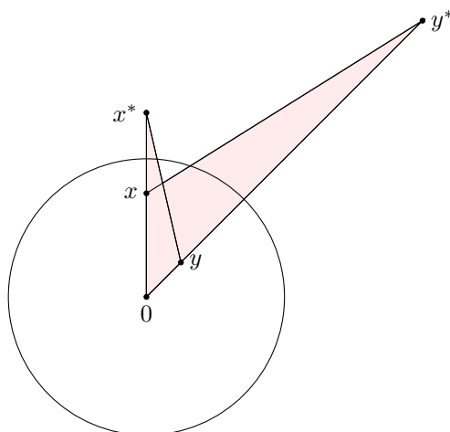
ABBILDUNG 1. Geometrischer Beweis von (iii): Die Dreiecke 0xy^* und 0yx^* sind ahnlich.
