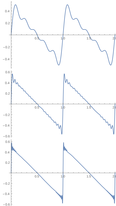
ABBILDUNG 2. Die N -te Partialsumme ( N = 5, 20, 50 ) der Fourierreihe der Funktion f(x) = 1/2 - x , x \in [0, 1) , 1-periodisch fortgesetzt
