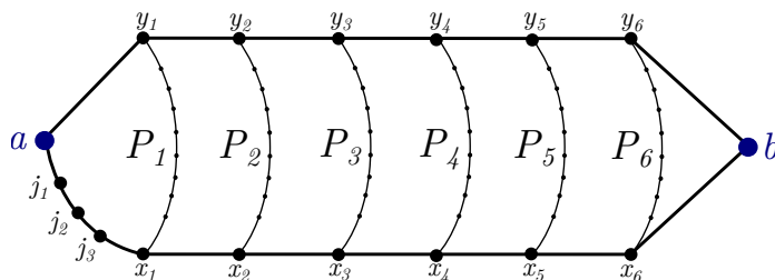
FIG. 1. A 3-gadget.
